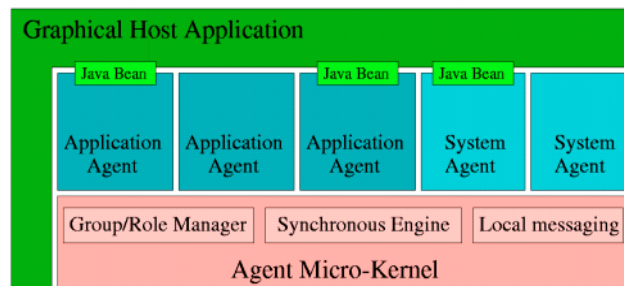
Figure 1. L'architecture générale de MadKit
